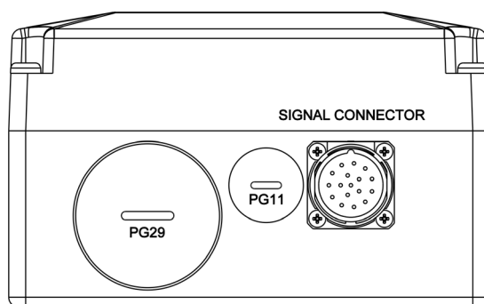
接线盒 142×142
